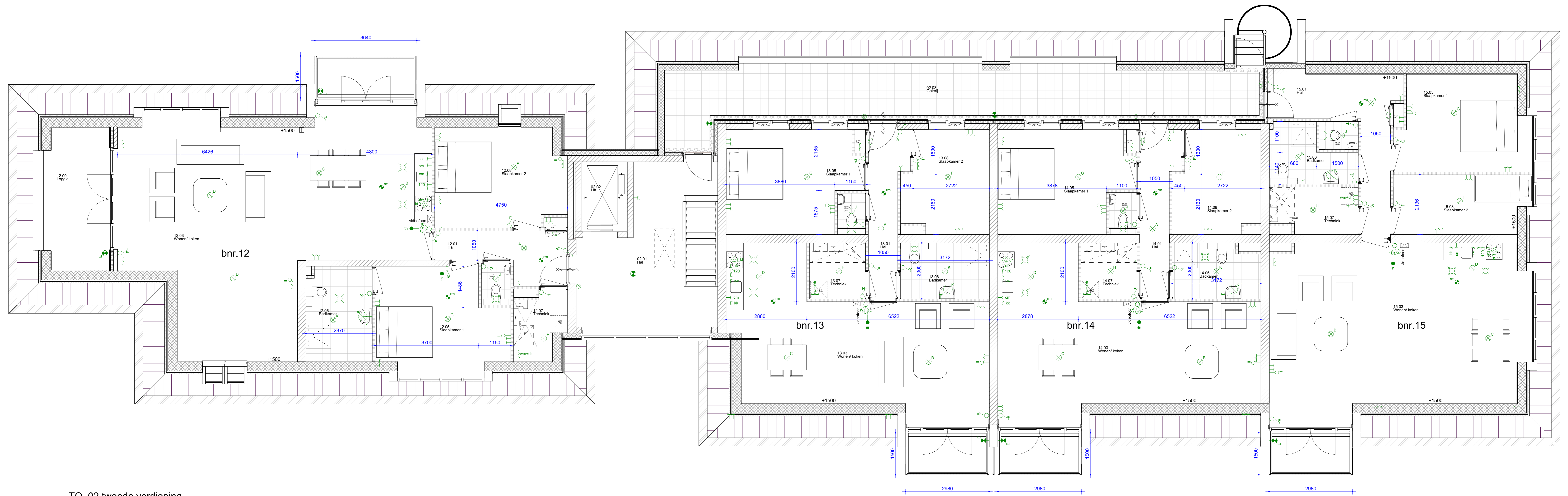
TO_02 tweede verdieping 1 : 50
